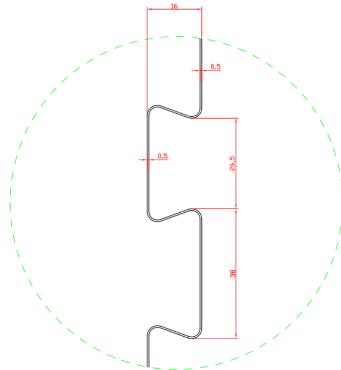
detalj i skala 2:1
